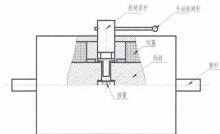
图2 电磁铁内部结构图
