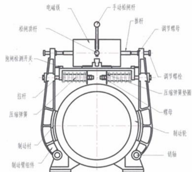
图1 鼓式制动器（双铁芯）
