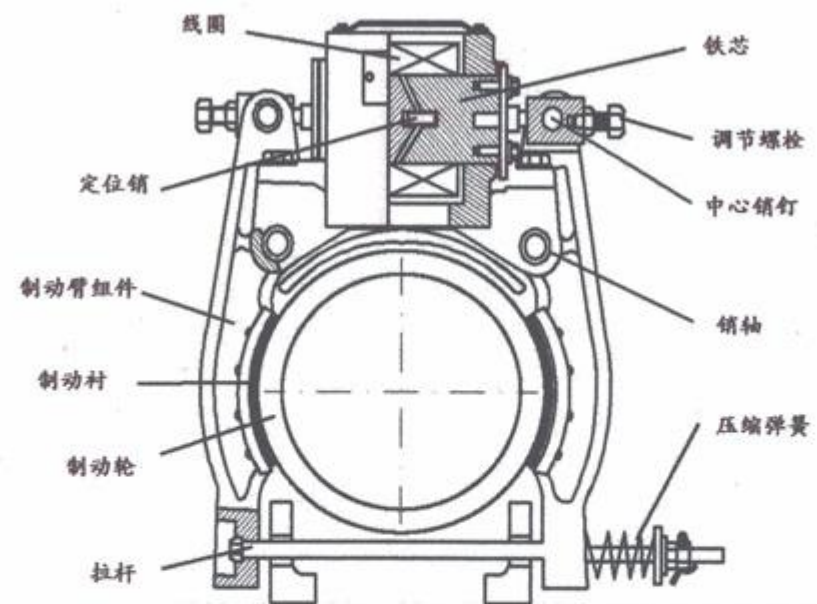
图 3 鼓式制动器（单铁芯）
